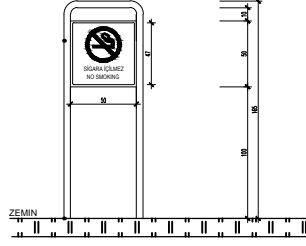
ÖN GÖRÜNÜŞ SİSTEM DETAYI Ö :1/20
