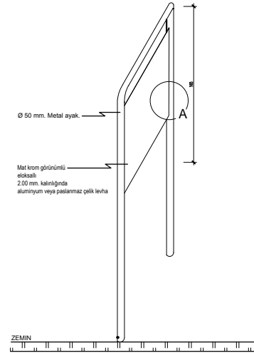
BAĞLANTI DETAYI
